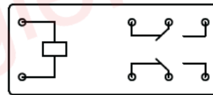
2转换 2C 型
